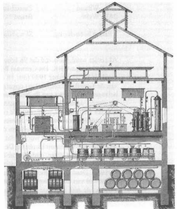
Dwarsdoorsnede van een brouwerij met koelinstallatie eind 19e eeuw.
